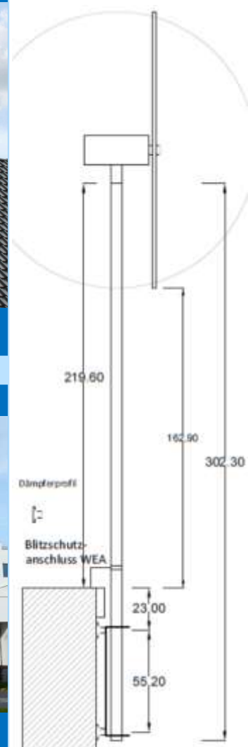
SkyWind Flanschmast
