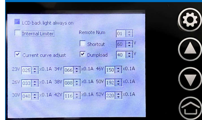
Das Einstellungs Menü des Wechselrichters (Beispiel)
