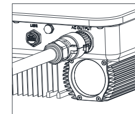
Abb. 6.4 AC-Schnellanschluss-Schema
