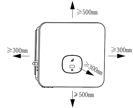
Abb. 5.2 Installationsdimensionen des Wechselrichters
