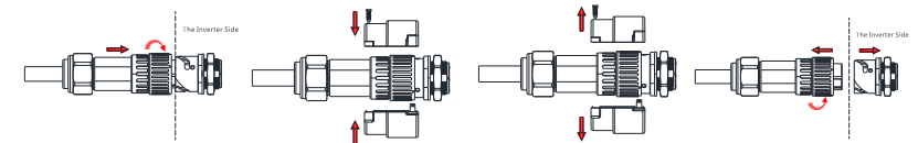
Abb. 6.3 Anschlusschema der AC-Klemme
