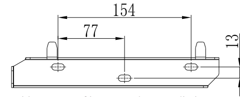
Abb. 5.7 Spezifikationen der Wandhalterung
