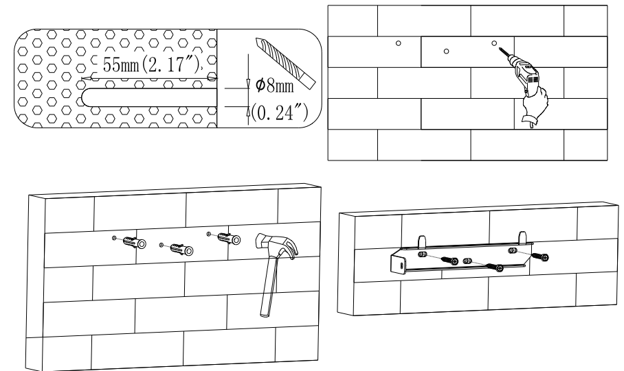
Abb 5.8 Schematische Darstellung der Wandmontage
