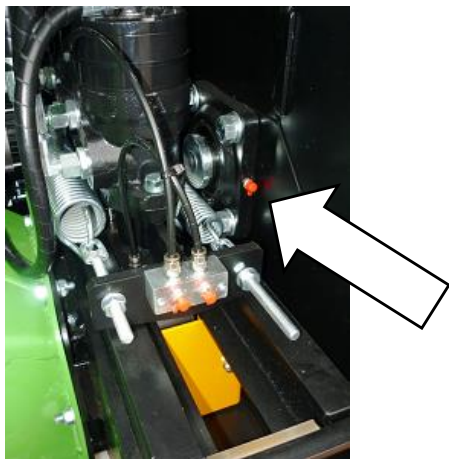
Schmierbüchsen an Lagerung der Zerkleinerungsscheibe
