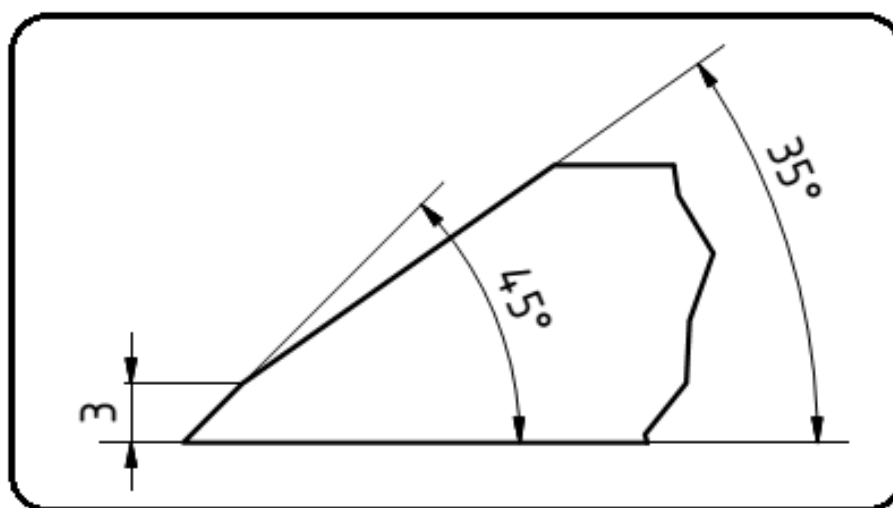
Schneidegeometrie der Messerschneide
