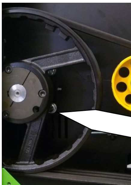
Anbringung des Drehzahlgebers unter der Haube
