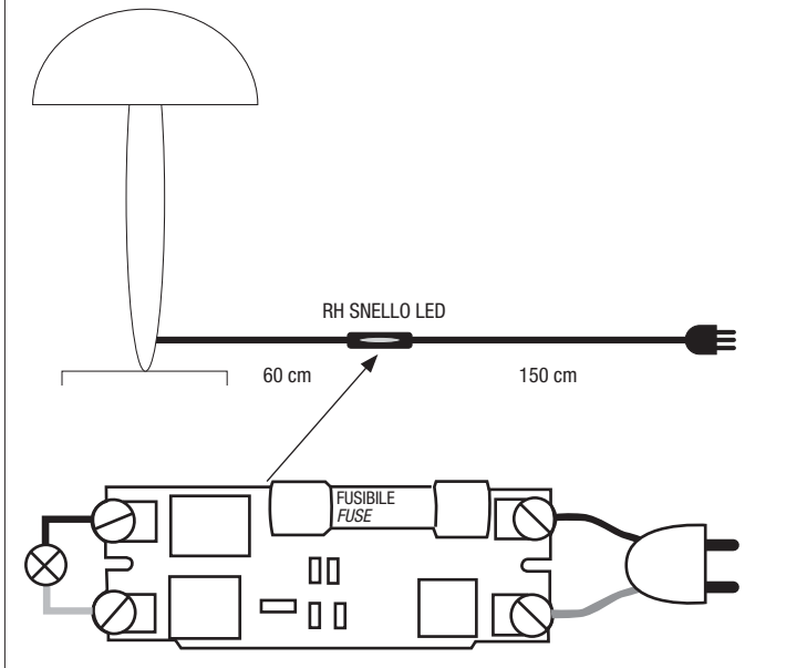
Fig. 2 - Cablaggio - Wiring - Verkabelung
