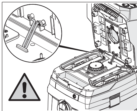
Рис. 77: Стопорная скоба
