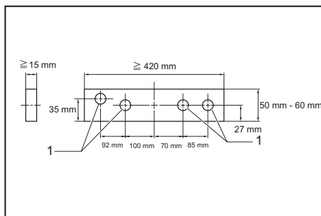
1. Agujeros
