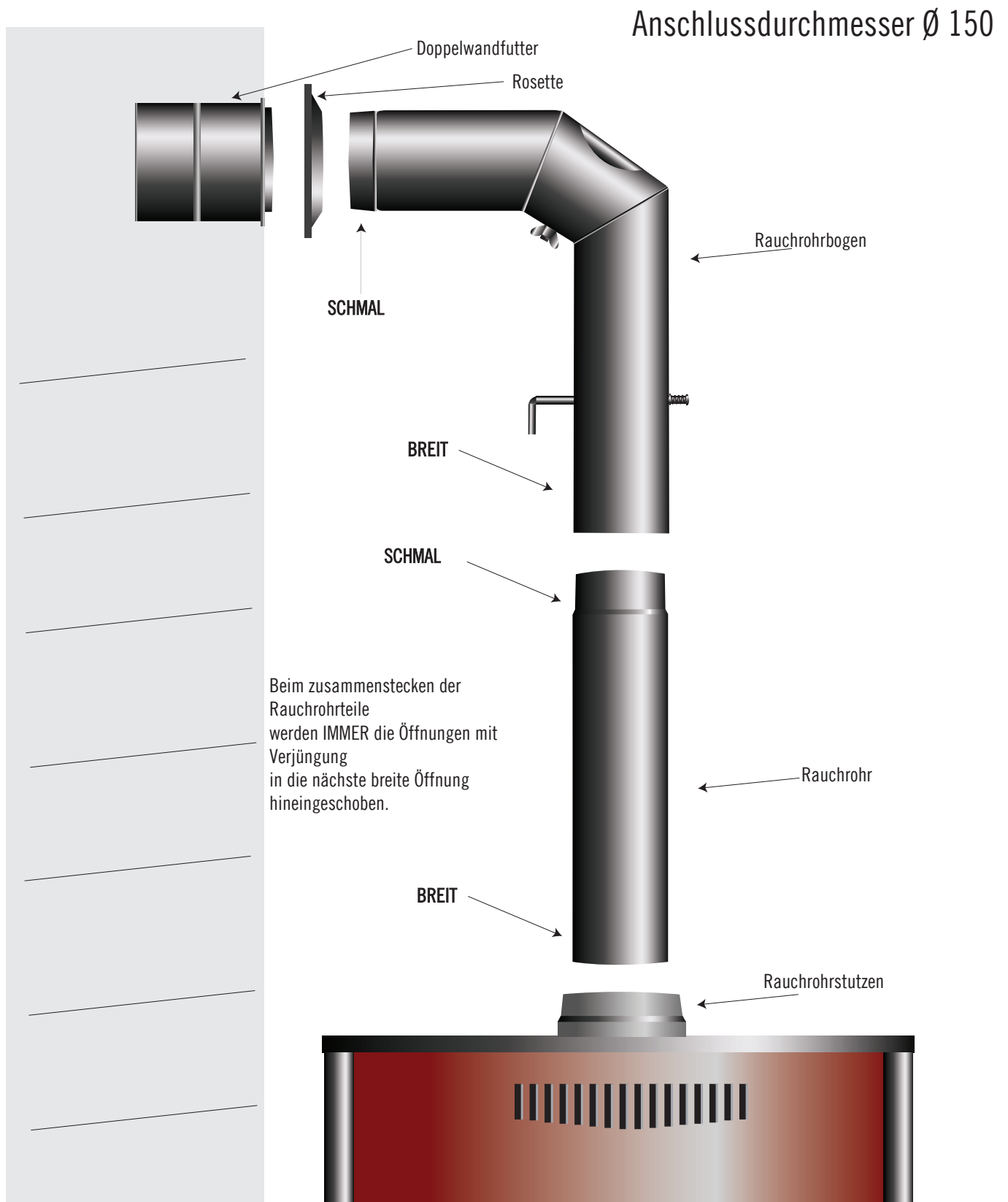
Abbildung 1 Rauchrohranschluss
