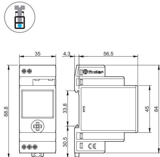
12.61 / 12.A1 Schraubklemmen
