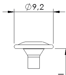
Rückwandkopf
