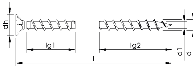
Unterkopfgewinde ohne Variation, ohne Schafttrippen, mit Spitzenverzahnung
