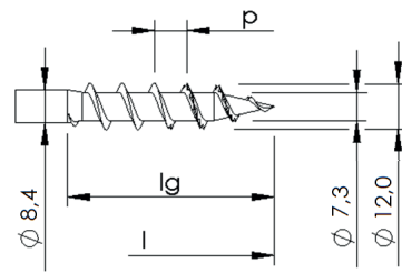
Mit und ohne Gewindevariation, mit Spitzenverzahnung
