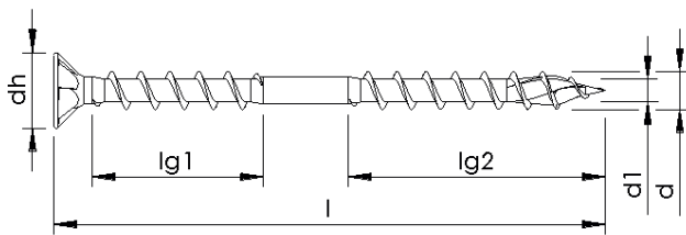
Unterkopfgewinde ohne Variation, ohne Schafttrippen, mit Spitzenrippen
