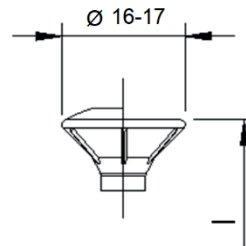
Flachsenkkopf mit und ohne Linse, mit und ohne Fräsrippen
