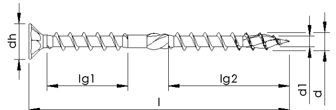
Unterkopfgewinde ohne Variation, mit Schafttrippen, Spitzenverzahnung und Spitzenrippen
