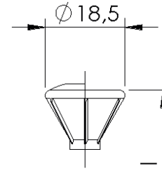
Flachsenkopf 60° / 75° mit und ohne Linse, mit und ohne Fräsrippen
