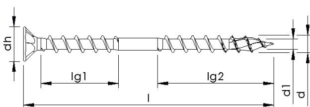
Unterkopfgewinde ohne Variation, ohne Schafttrippen, mit Spitzenverzahnung und Spitzenrippen
