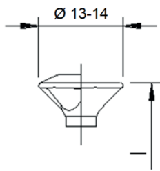
Flachsenkkopf mit und ohne Linse, mit und ohne Frästaschen
