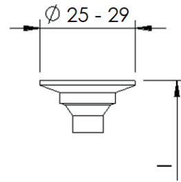
Flachtellerkopf mit und ohne Fräsrippen
