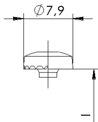
Panhead mit und ohne Unter- kopffräsrippen
