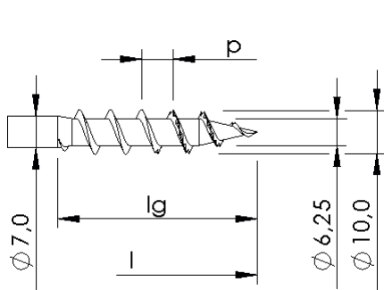
Mit und ohne Gewindevariation, mit Spitzenverzahnung
