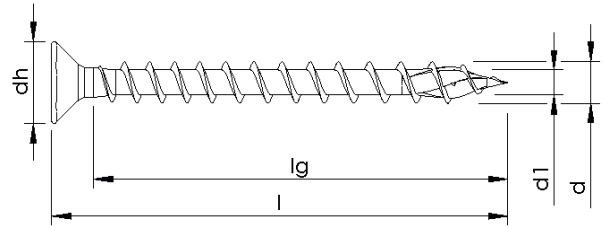
Vollgewinde mit Variation, mit Spitzenrippen
