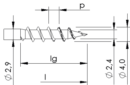
Mit und ohne Gewindevariation, mit Spitzenverzahnung
