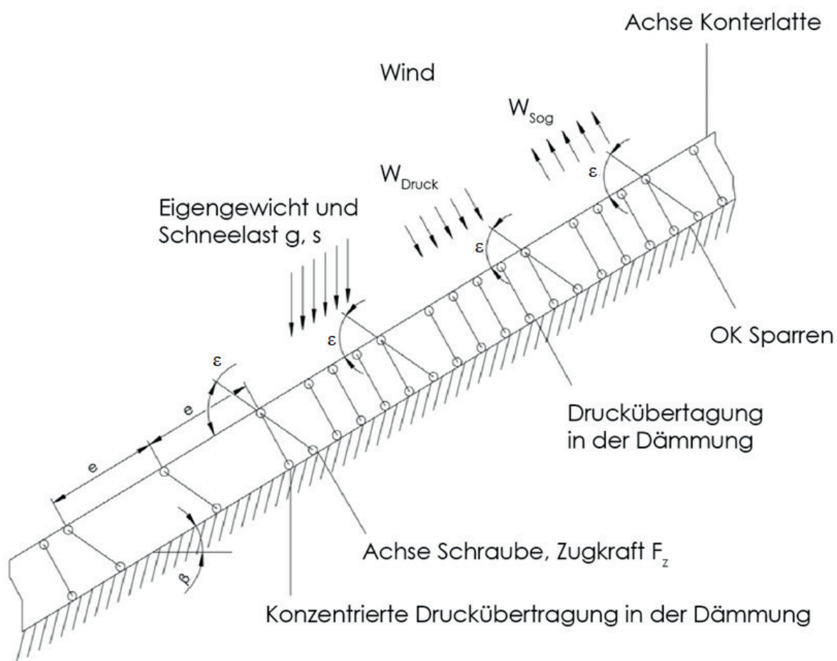
Abbildung 7: Befestigung von Aufdach-Dämmsystem-Bauweise mit parallel geneigten Schrauben
