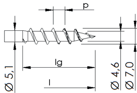
Ohne Gewindevariation, mit Spitzenverzahnung
