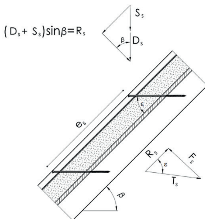
Abbildung 9: Einzellasten F_s rechtwinklig zu den Latten, Lastangriff im Bereich der Schraubenköpfe
