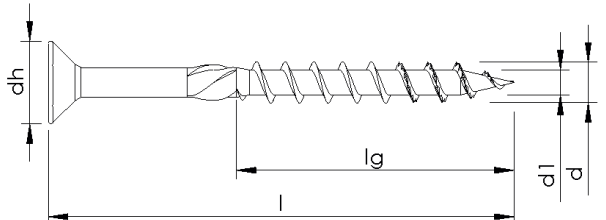
Teilgewinde ohne Variation, mit Schaftrippen und Spitzenverzahnung
