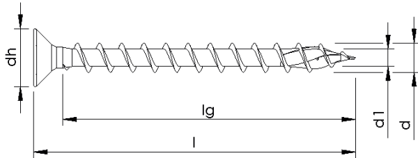
Vollgewinde ohne Variation, mit Spitzenrippen
