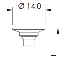
Flachtellerkopf mit und ohne Fräsrippen
