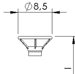
Flachsenkopf mit und ohne Fräsrippen
