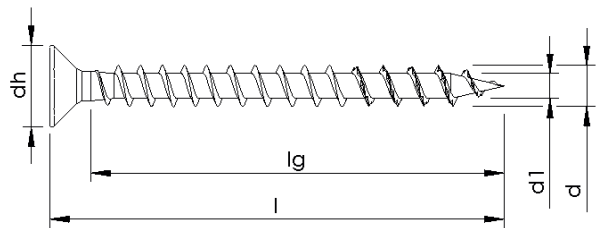
Vollgewinde mit Variation, mit Spitzenverzahnung
