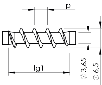
Unterkopfgewinde
