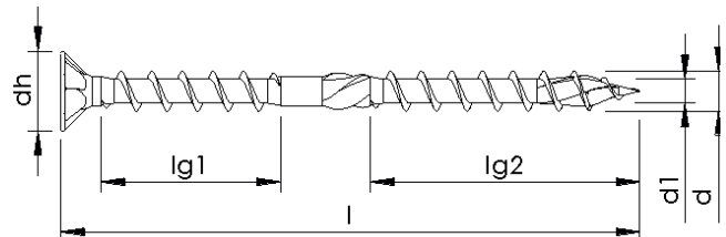
Unterkopfgewinde ohne Variation, mit Schafttrippen und Spitzenrippen
