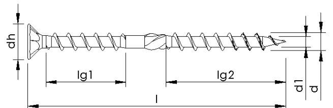
Unterkopfgewinde ohne Variation, mit Schafttrippen und Spitzenverzahnung
