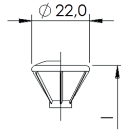
Flachsenkopff 60° / 75° mit und ohne Linse, mit und ohne Fräsrippen
