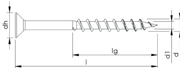
Teilgewinde ohne Variation, ohne Schaftrippen, mit Spitzenverzahnung
