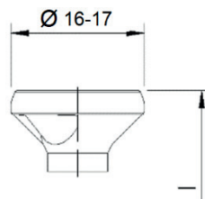
Flachsenkopf, mit und ohne Frästaschen
