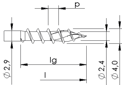
Mit und ohne Gewindevariation, mit Spitzenrippen
