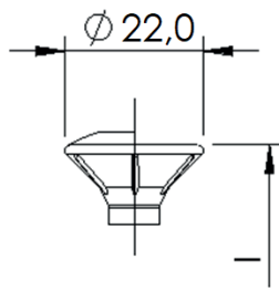
Flachsenkopff mit und ohne Linse, mit und ohne Fräsrippen
