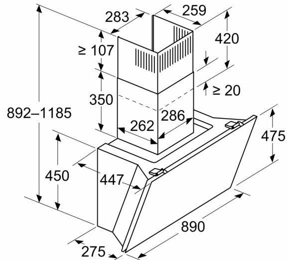
Maße in mm Gerät im Umluftbetrieb
