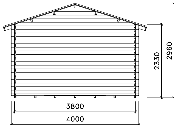
Schnitt A-A
