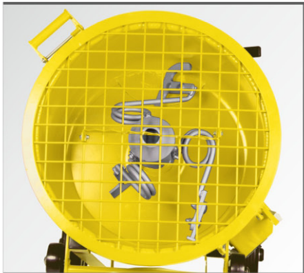
Die drei Mischarme verarbeiten das Material gründlich. Die Wand- abstreifer verhindern Mischgutab- lagerungen an der Trommelwand.
