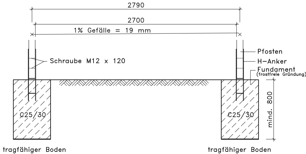
Schnitt B-B
