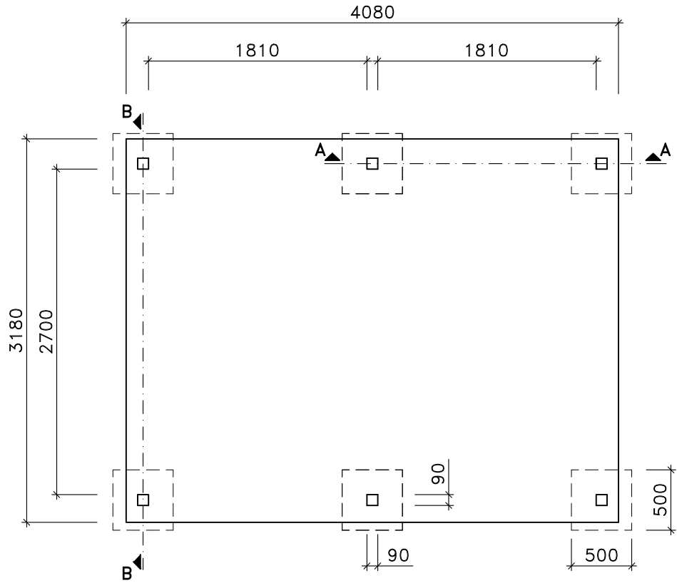
Grundriß
