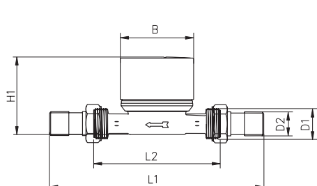
Abmessungen
