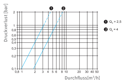
Druckverlustkurve
