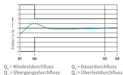
Typische Fehlerkurve
