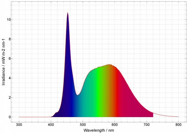
Spektrale Lichtverteilung:
