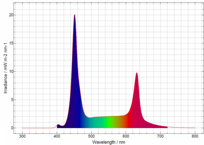
Spektrale Lichtverteilung:
