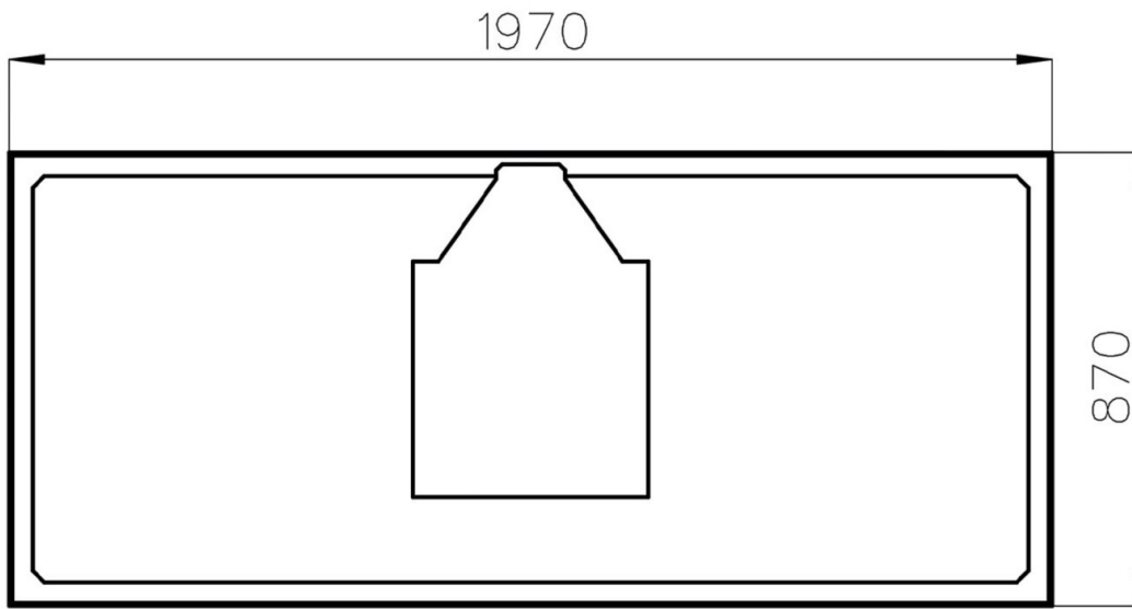
Draufsicht
