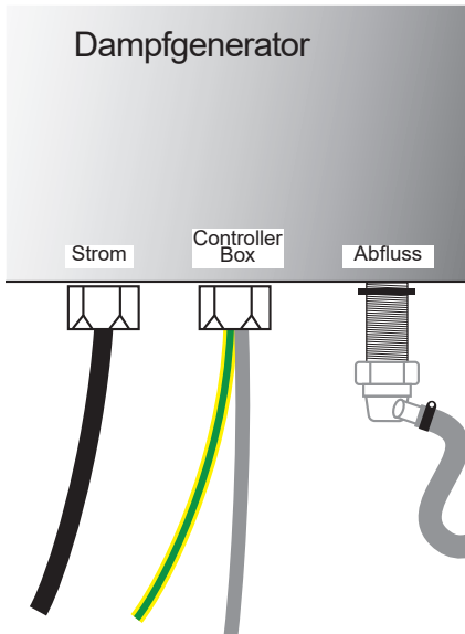
Abbildung zeigt den Anschluss des Ablaufes an den Dampfgenerator.
