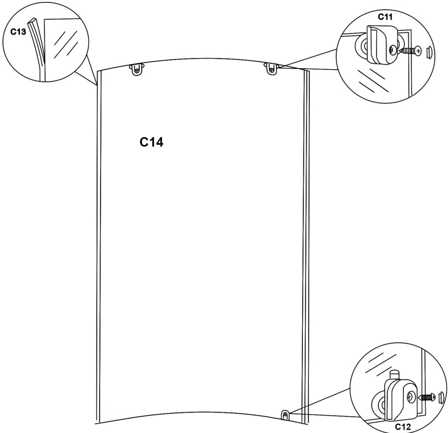
Türdichtung, F-Dichtung
