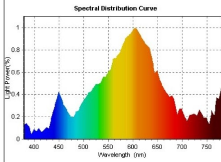
光谱分布
