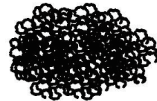
B(lava rocks)
