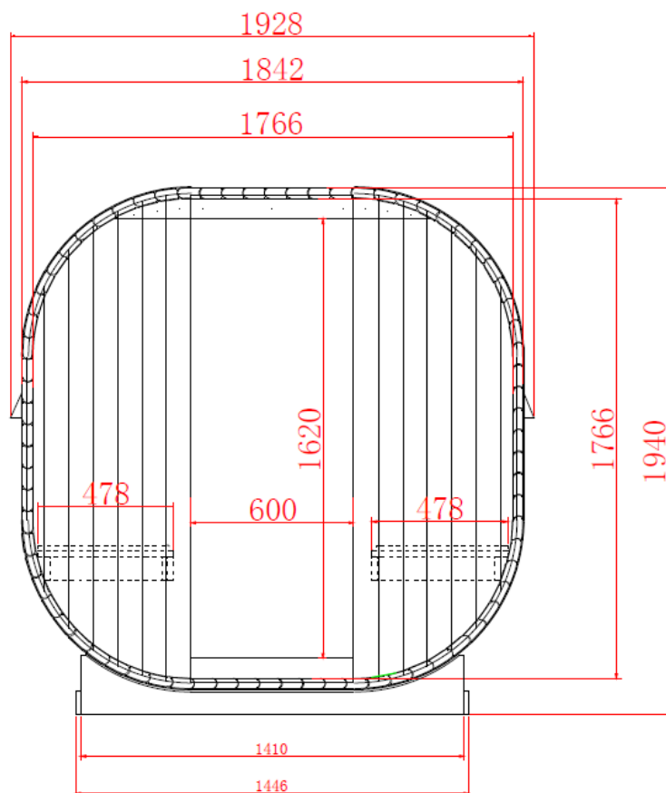
Abbildung 3 Skizze Cube M Frontansicht mit Maßen in mm
