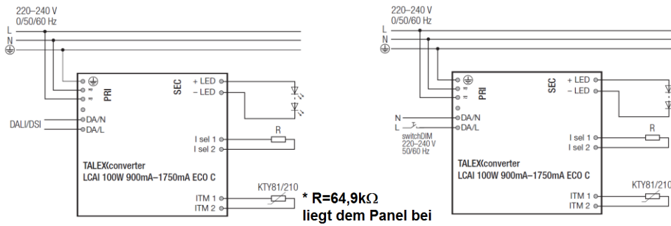
Anschlussdiagramm
