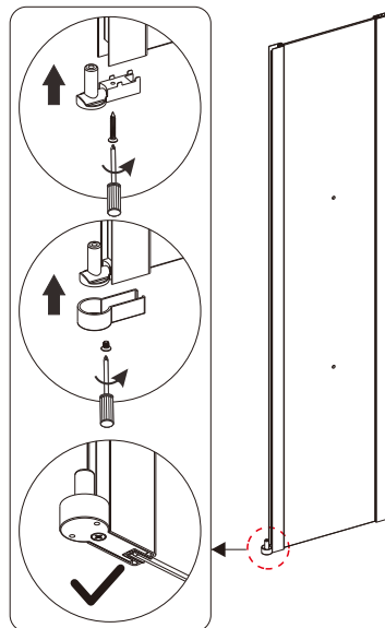
Anschlag rechts
