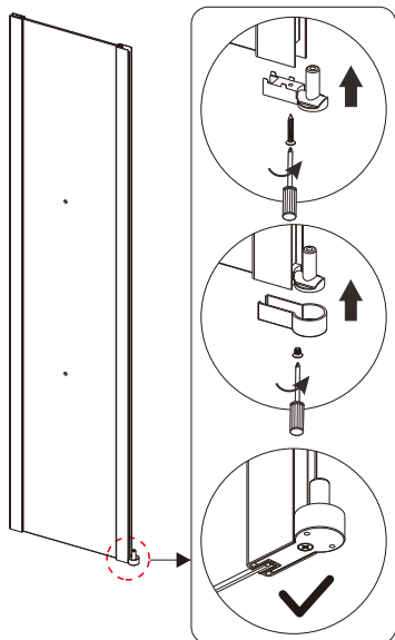
Anschlag links
