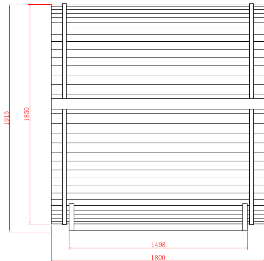
Abbildung 2 Skizze Lahti M Seitenansicht mit Maßen in mm
