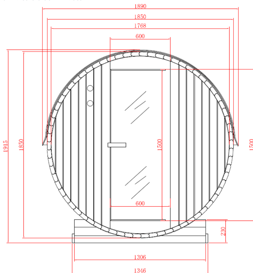
Abbildung 3 Skizze Lahti L Frontansicht mit Maßen in mm
