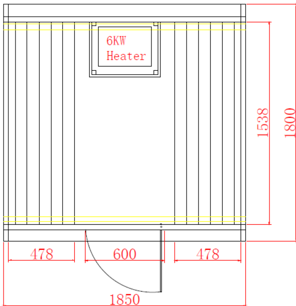
Abbildung 4 Skizze Lahti L Innenraumansicht mit Maßen in mm
