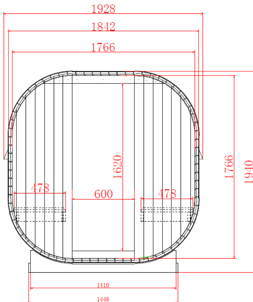
Abbildung 3 Skizze Cube XL Frontansicht mit Maßen in mm
