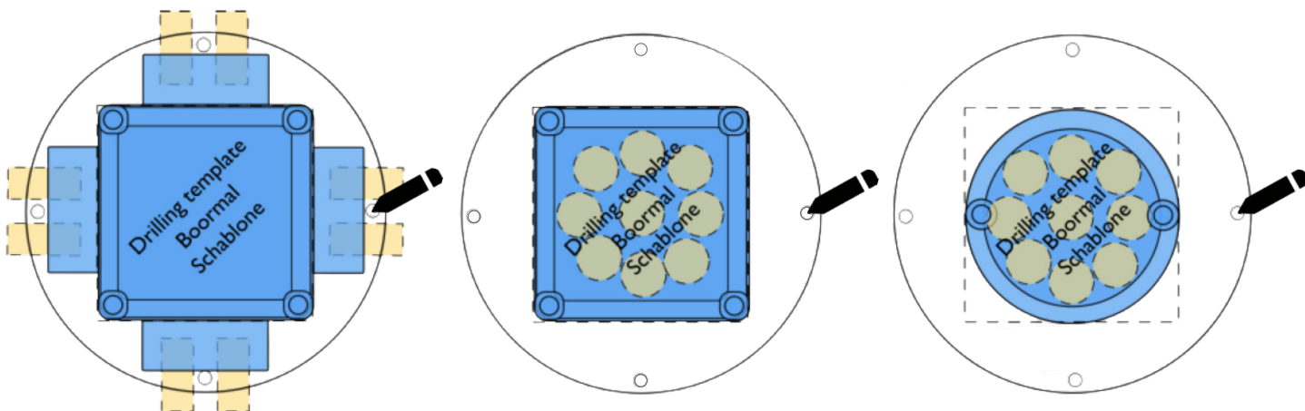
Verteilerdose (Gips)
