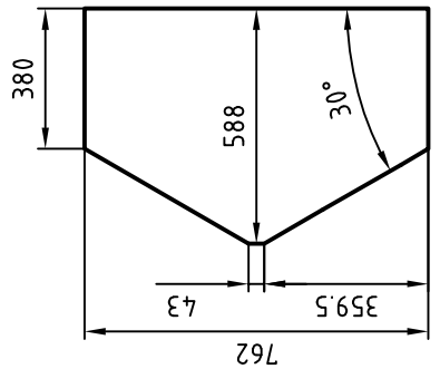
Detail Y
