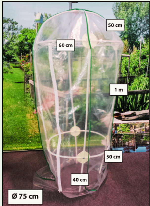
Img.6) Limonaia diam. 120cm & 75cm con misure / Frostschutzhaube Diam. 120cm & 75cm mit Maße
