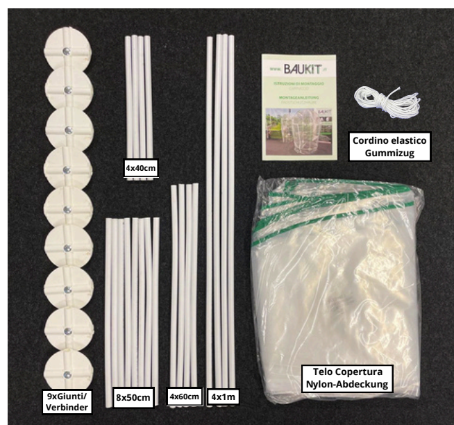
Img.2) Limonaia/Frostschutzhaube Ø 75cm
