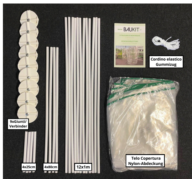
Img.1) Limonaia/Frostschutzhaube Ø 120cm
