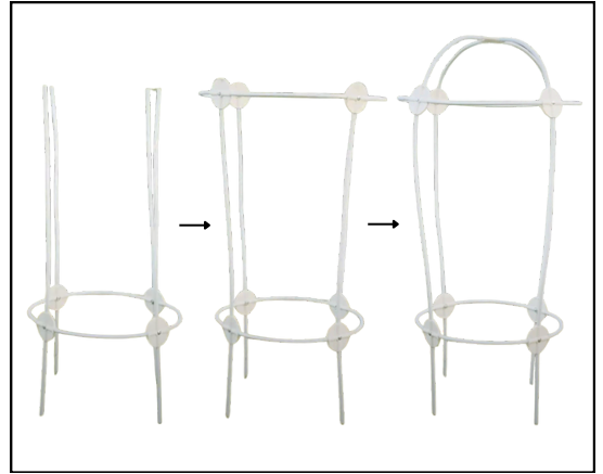
Img.5) Piegatura tubi & Completamento struttura limonaia / Biegung der Rohre & Fertigstellung der Struktur der Haube
