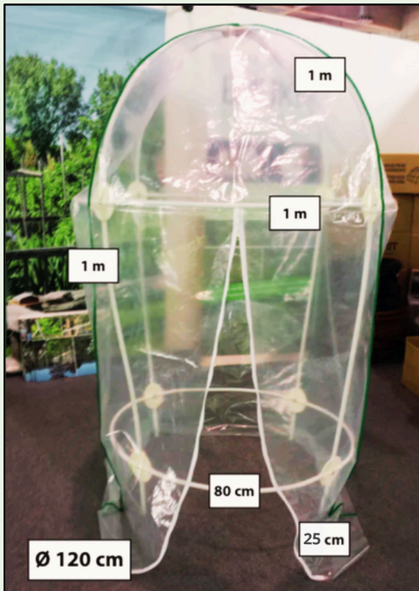
Img.6) Limonaia diam. 120cm & 75cm con misure / Frostschutzhaube Diam. 120cm & 75cm mit Maße
