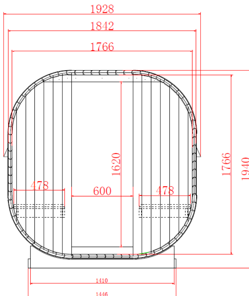
Abbildung 3 Skizze Cube L Deluxe Frontansicht mit Maßen in mm
