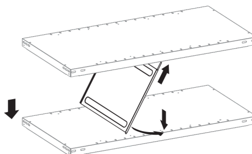
Abb. 3 Einsatz der Tennbleche
