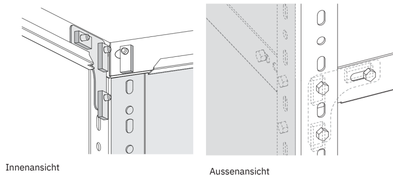
Abb. 2 Verschraubung der Eckplatten
