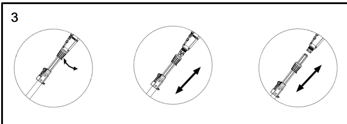
Rysunek 3: Demontaż silnika z głowicą tnącą z zawieszenia teleskopowego w celu zaoszczędzenia miejsca podczas przechowywania lub transportu.
