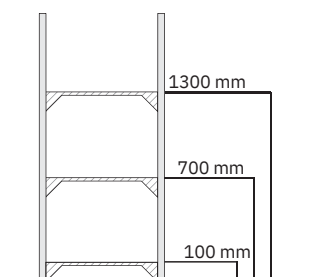
Abb. 15 Anordnung vordere Traverse Disposition des longerons avant Plaatsing dwarsbalk aan de voorzijde Arrangement of the front cross-arm
