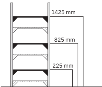
Anordnung hintere Traverse Disposition des longerons arrière Plaatsing dwarsbalk aan de achterzijde Arrangement of the rear cross-arm
