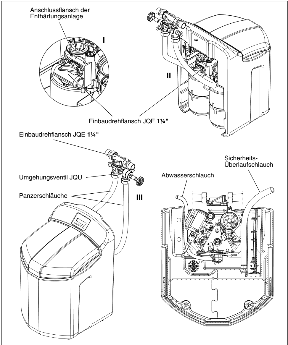
Abb. 6: Montage der Enthärtungsanlage
