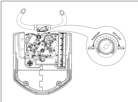
Abb. 11: Einstellen der Verschneidung
