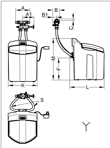
Abb. 18: Einbaumaße
