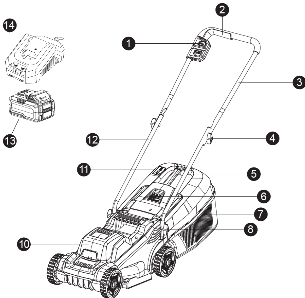
Ilustración: Cortadora de césped
