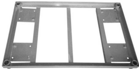
Bodenplatte A
