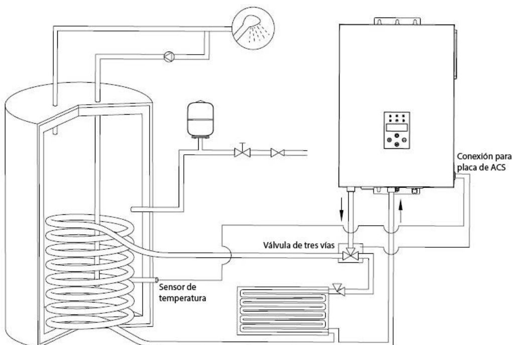
Esquema de la instalación completada para la función ECS
