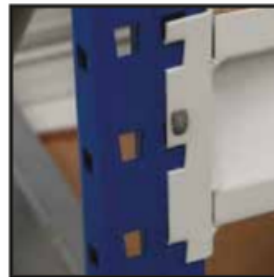
Längsträger und Sicherheitsstifte befestigung
