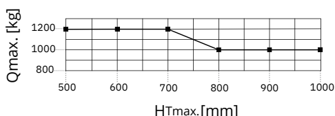
Abb. 12 Feldlasten für Regalhöhe: Charges de travée pour une hauteur d'étagère: Veldbelastingen voor stellinghoogtes: Bay loads for a rack height:
