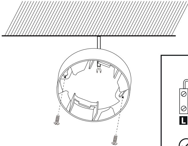
Schritt 1: Die Abdeckung befestigen
