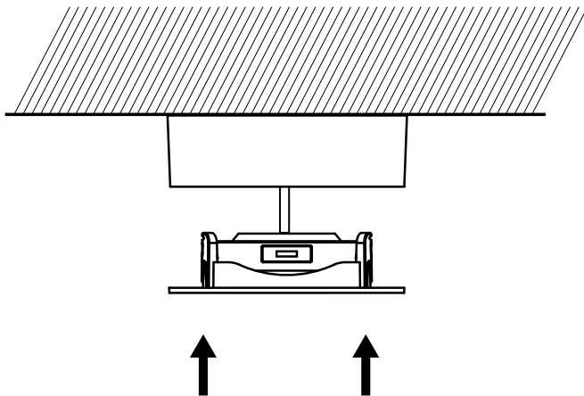
Schritt 3: Die Lampe in die Abdeckung einsetzen
