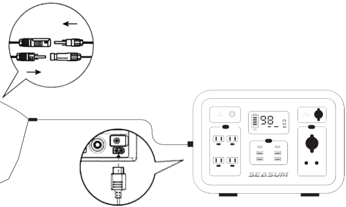
Collegare il cavo di ricarica
