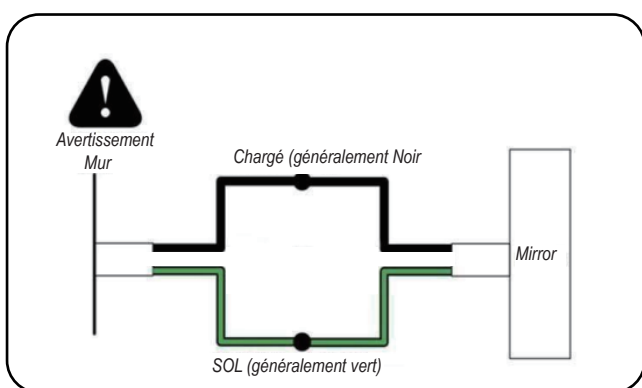
5. Conecte el espejo con el suministro principal.
